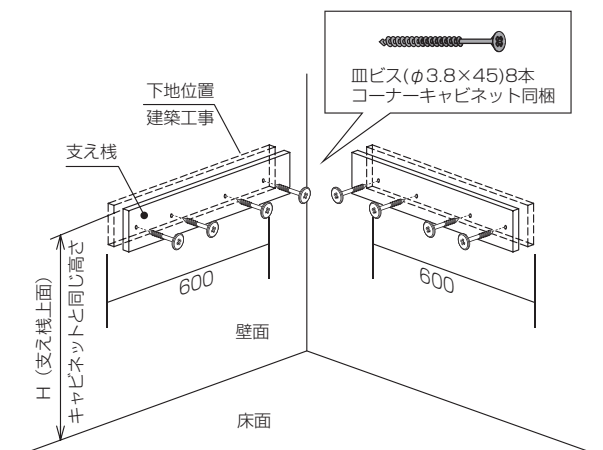
桟の取り付け高さ
