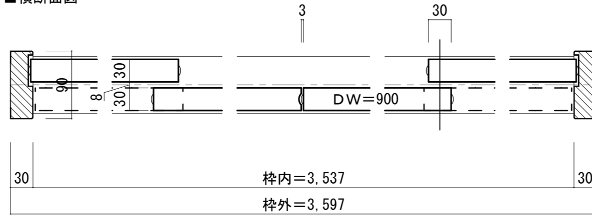
■横断面図
