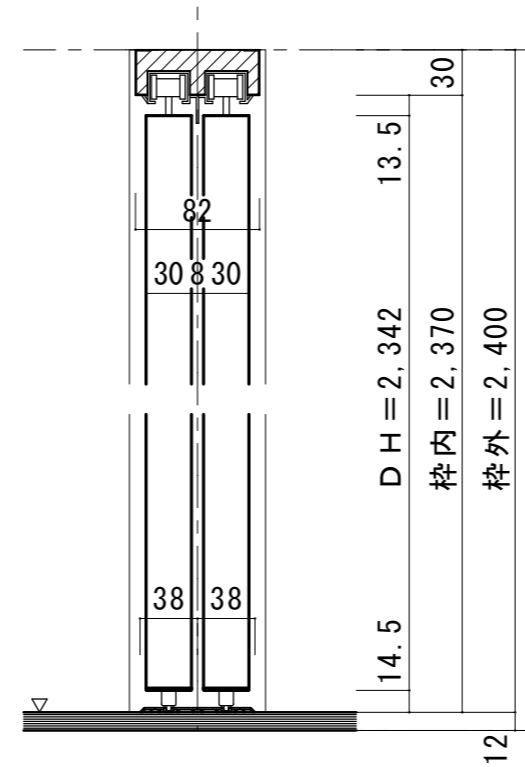
■縦断面図
