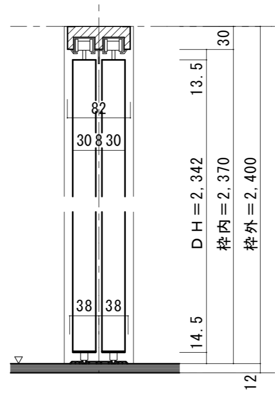
■縦断面図
