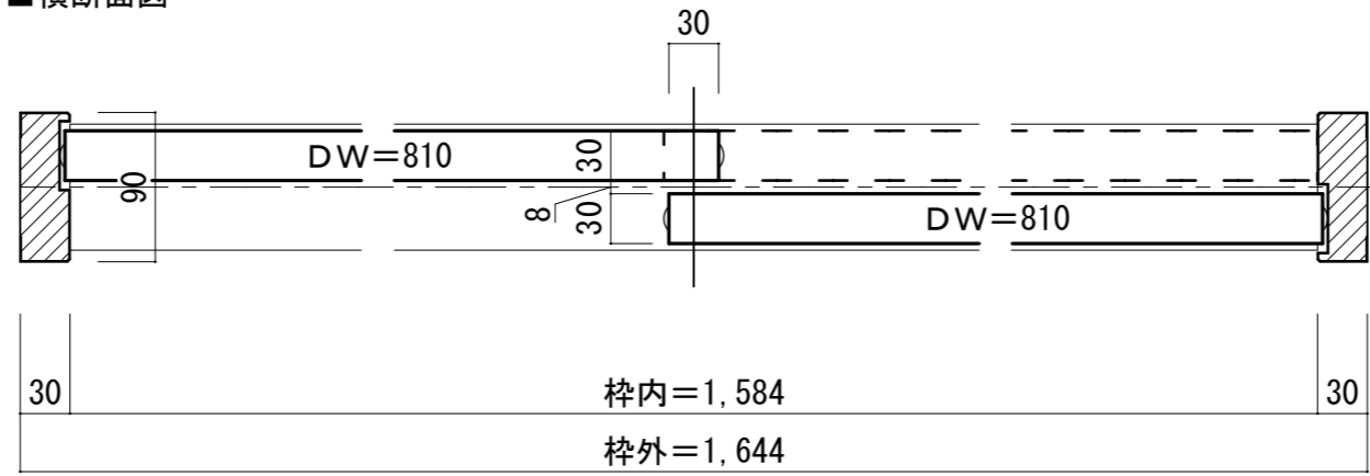
■横断面図
