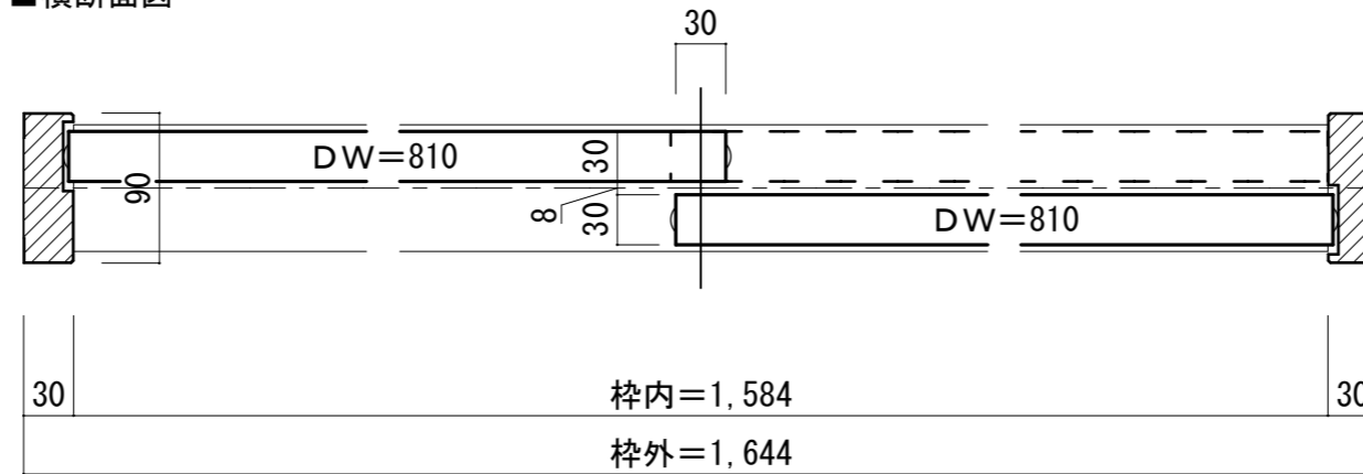
■横断面図
