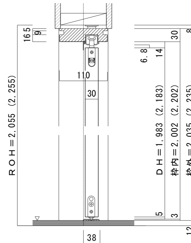
■縦断面図 [床直付けレールタイプ]
