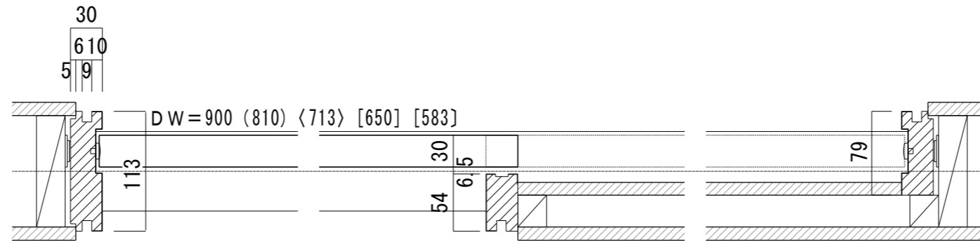
■横断面図
