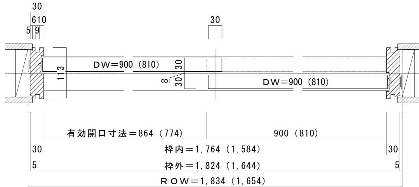
■横断面図
