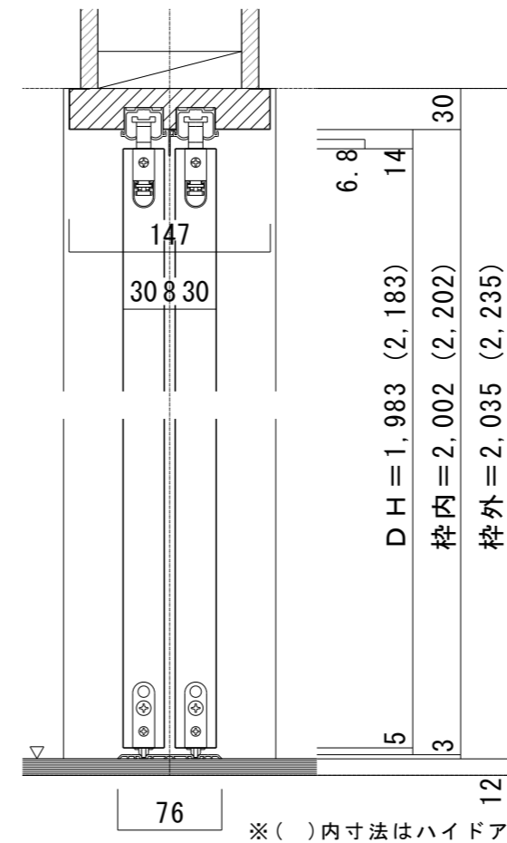
■縦断面図[床直付けルールタイプ]
