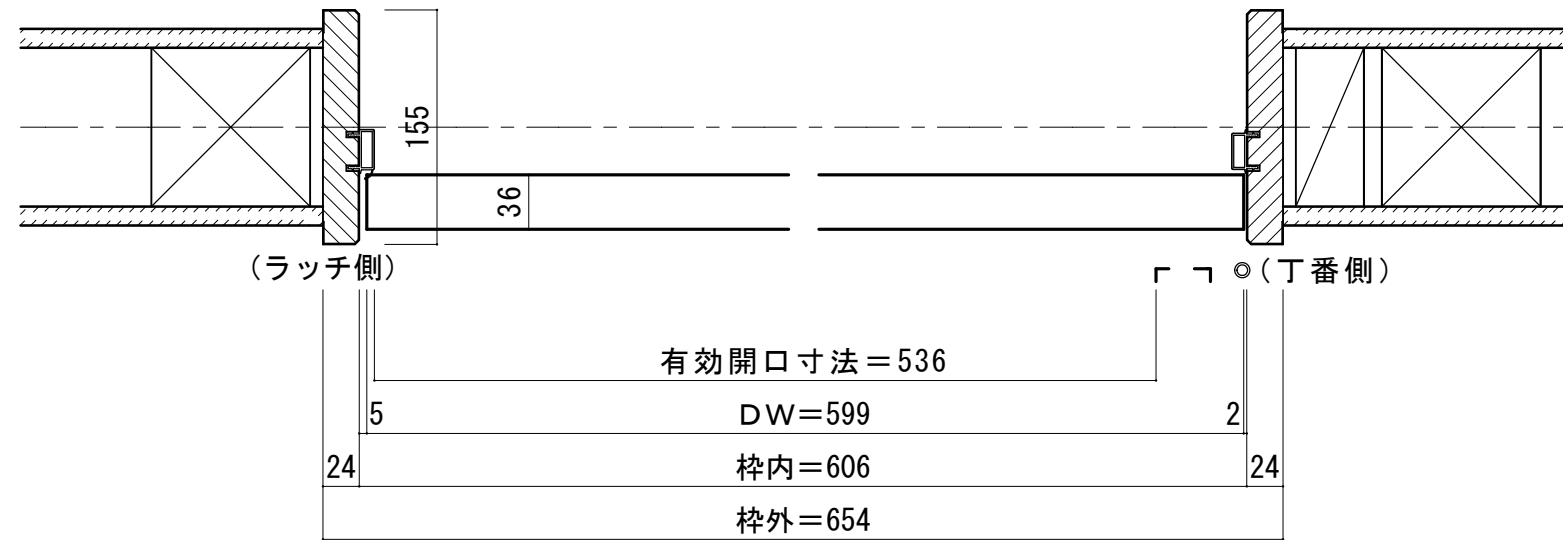
■横断面図
