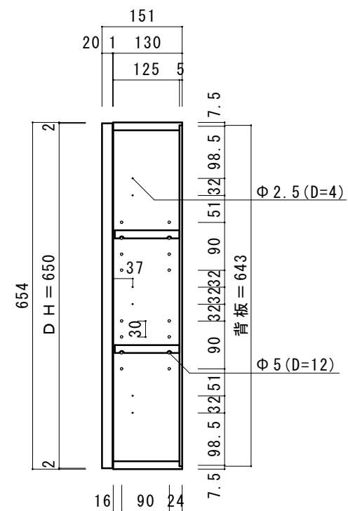
断面図
