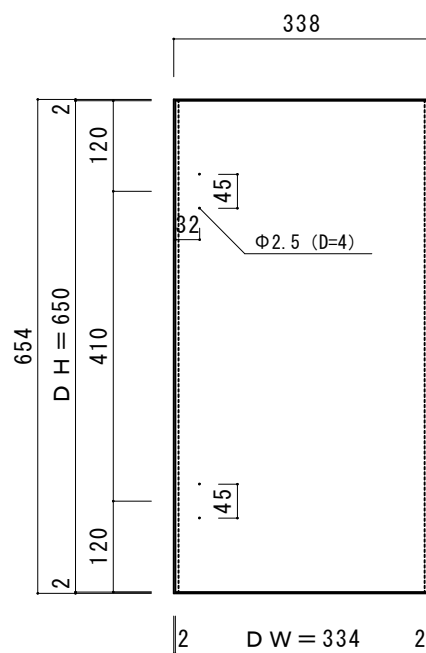
扉正面図
