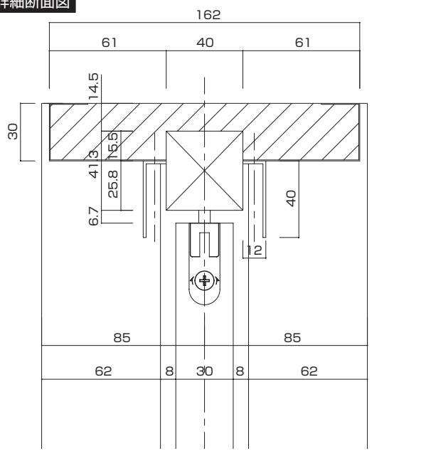
鴨居詳細断面図
