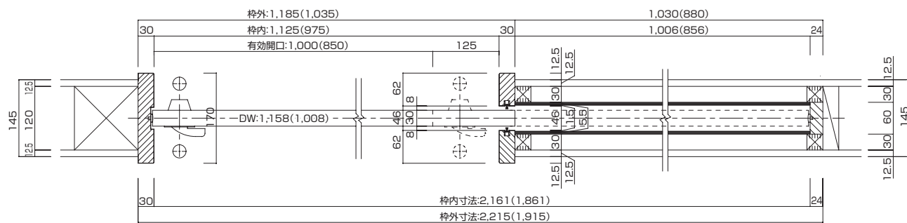
■レール詳細図
