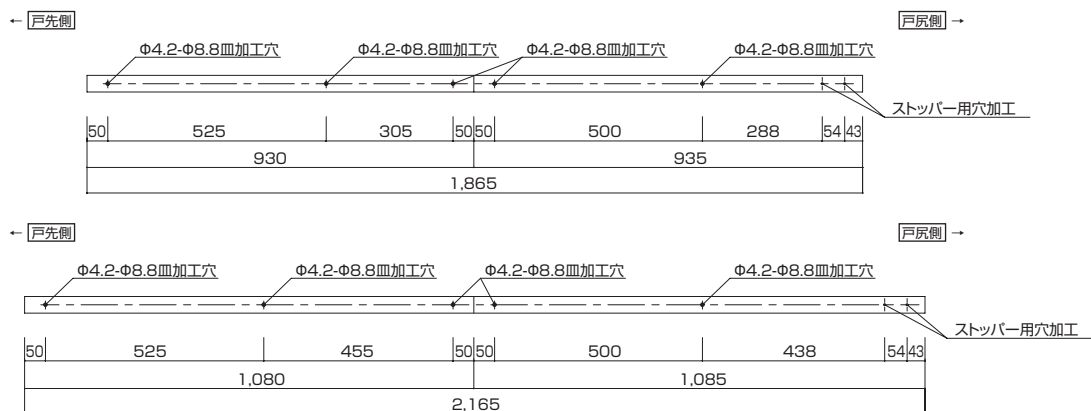
■レール詳細図
