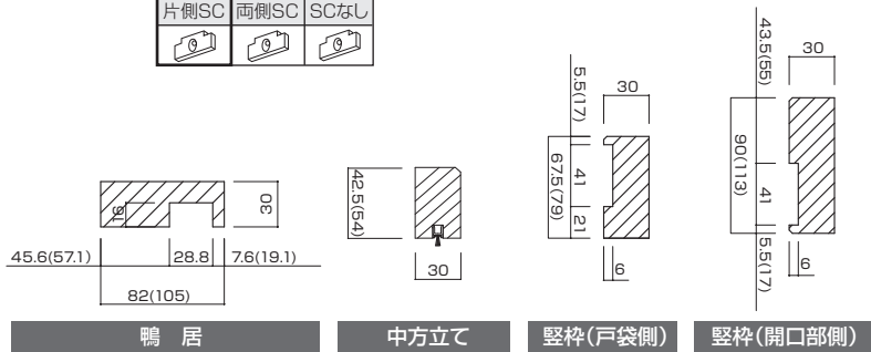
縦断面図
