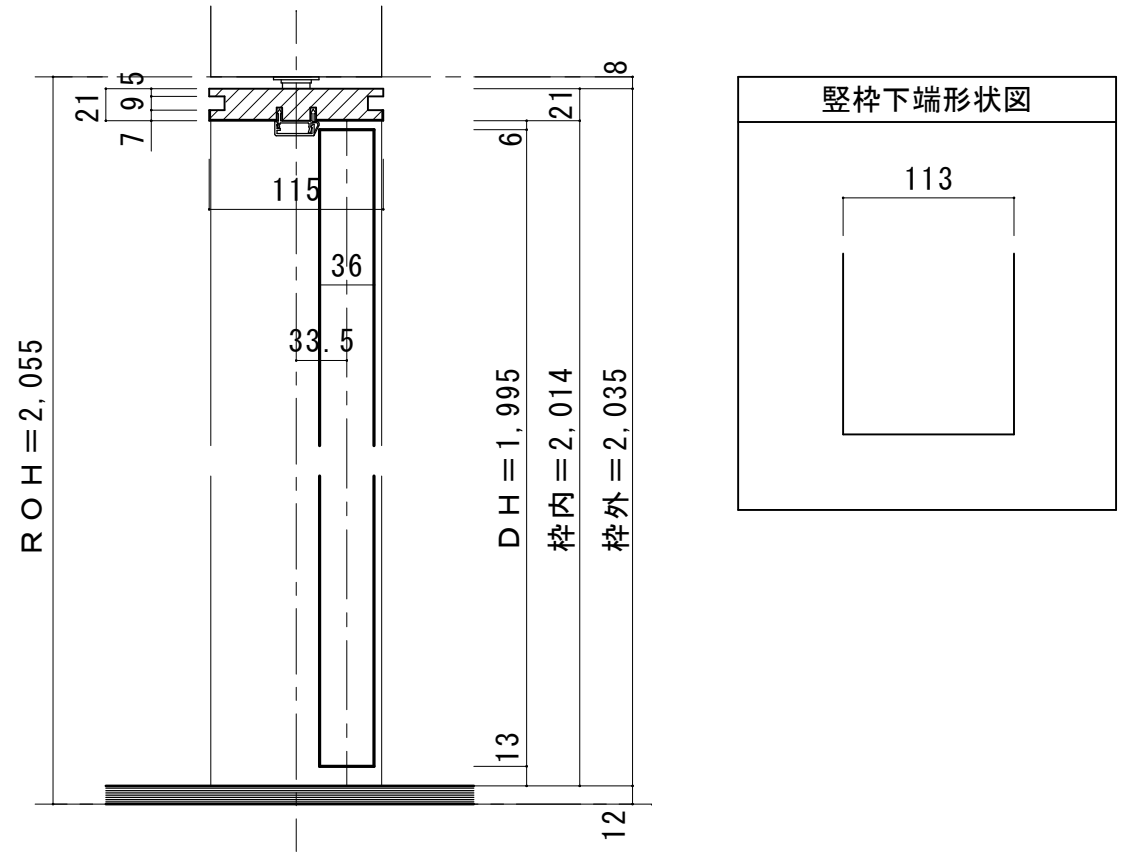
■ 縦断面図
