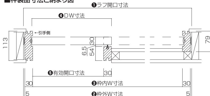
横断面図
