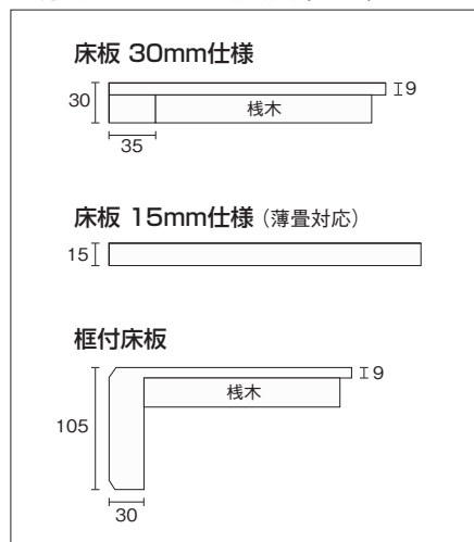
●樺・松シリーズ断面図(mm)
