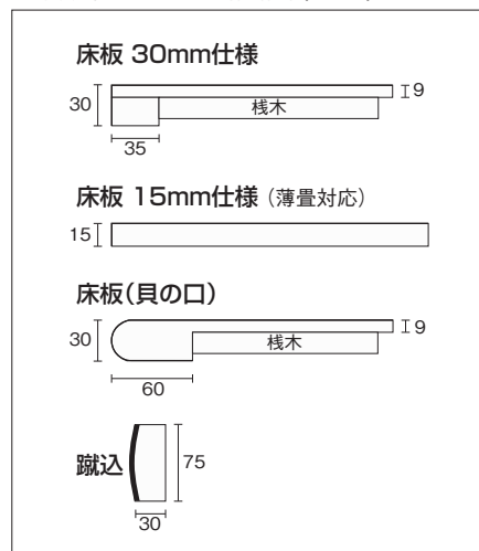
●春慶シリーズ断面図(mm)
