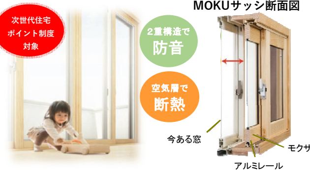
MOKUサッシ断面図
