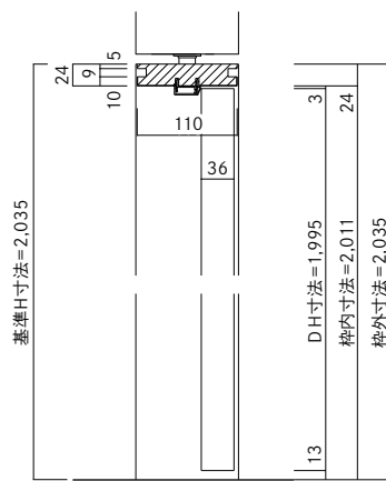
縦枠下端加工図
