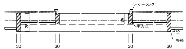
引き分け戸(和側引き込み)
