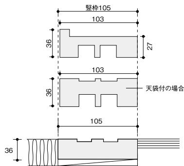
押し入れ引き違い戸枠セット
