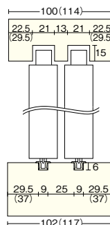
■真壁用 引き違い戸 納まり図寸法図(mm)
