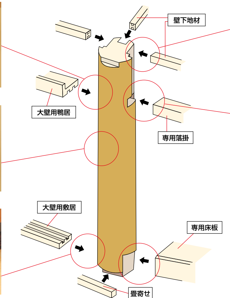
壁下地材との取り付け
