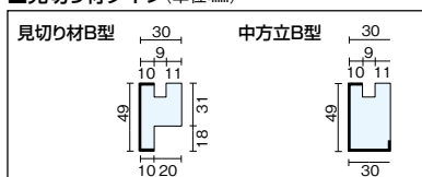
■ケーシング寸法・形状図(単位:mm)
