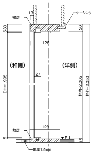
畳厚12mmご使用时(バリアフリー対応)敷居厚15mmタイプ (単位:mm)
