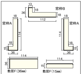
●正寸プレカット対応寸法図(mm)
