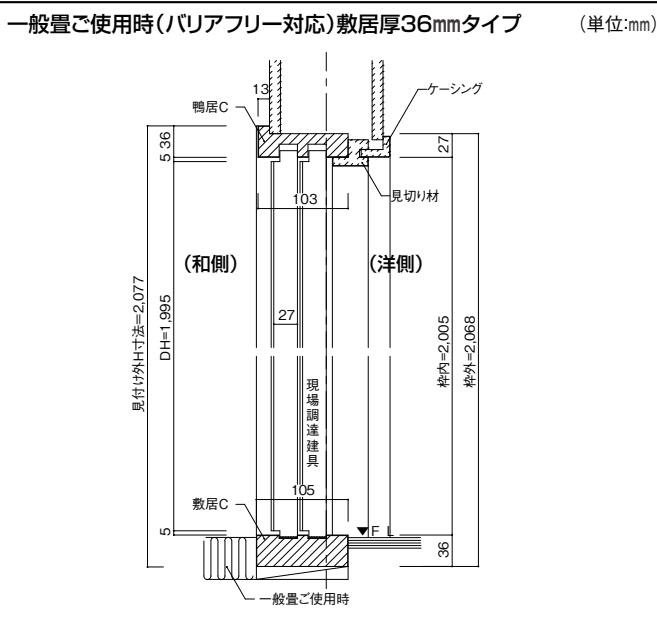
縦断面図
