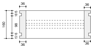
障子用(壁厚130mm限定) (単位:mm)
