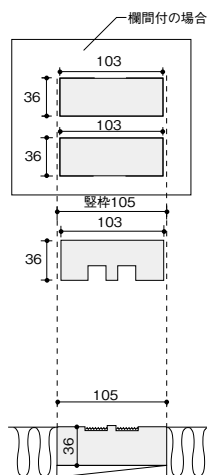
鴨居(無目)拡大図
