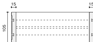
襖用(在来工法用) (単位:mm)
