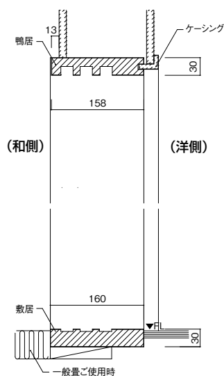
一般畳ご使用時(バリアフリー対応)敷居厚30mmタイプ
