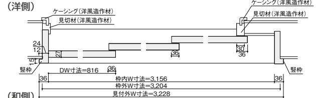
3枚引き込み戸(和側引き込み)
