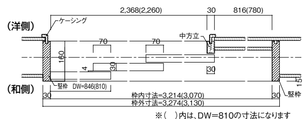
3枚引き込み戸(和側引き込み)
