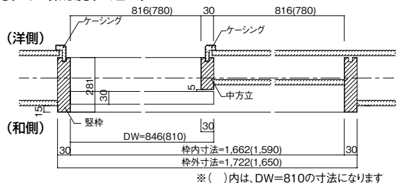
片引き戸(和側引き込み) (単位:mm)
