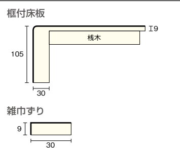
●断面図 (単位:mm)
