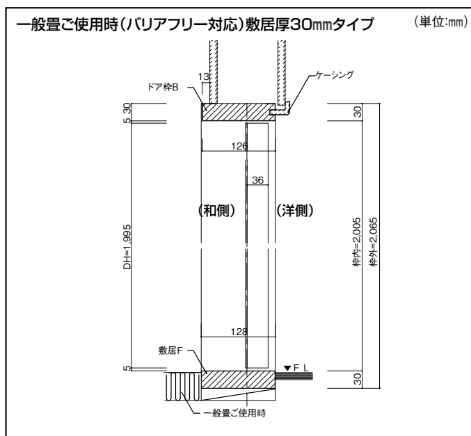
縦断面図
