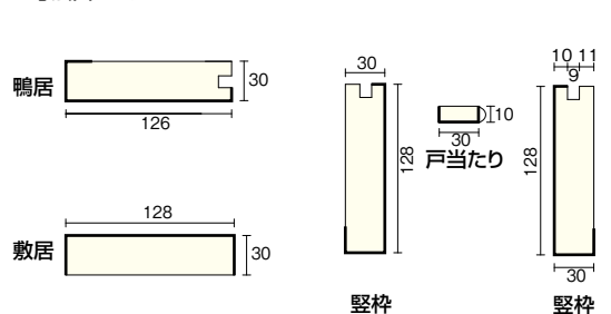
■寸法図 太線部分は化粧面
