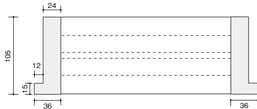
押し入れ引き違い戸枠セット
