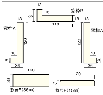
●在来工法用(窓枠幅120mm用)寸法図(mm)
