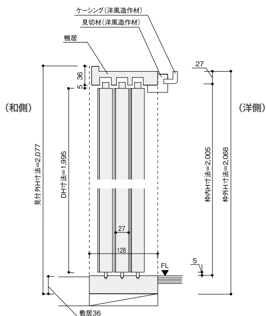
一般畳ご使用時(バリアフリー対応)敷居厚36mmタイプ
