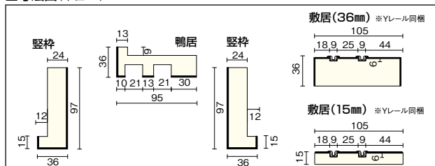
■寸法図(単位:mm)
