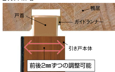
■オリジナル戸首
