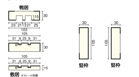
■寸法図 太線部分は化粧面
