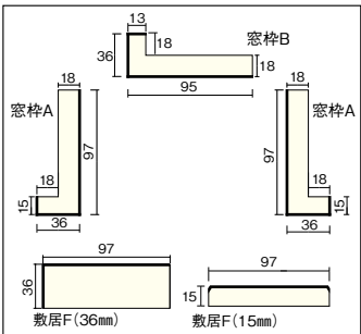
●2×4工法用寸法図(mm)
