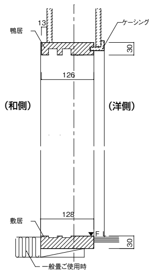
一般量ご使用时(バリアフリー対応)敷居厚30mmタイプ
