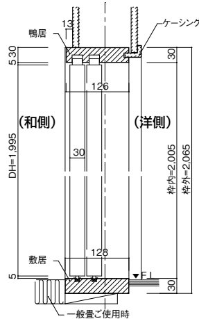
一般畳ご使用时(バリアフリー対応)敷居厚30mmタイプ
