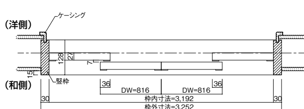
引き違い戸(12尺)
