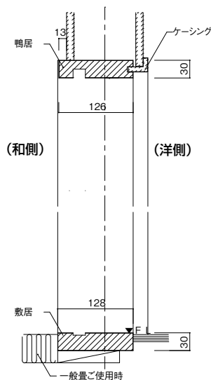
一般量ご使用時(バリアフリー対応)敷居厚30mmタイプ
