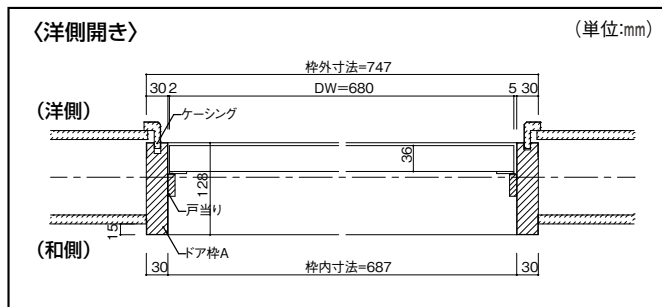
横断面図
