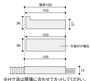
敷居寸法図
