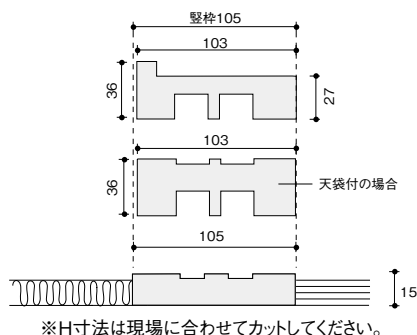
敷居寸法図
