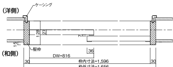
引き違い戸(6尺)
