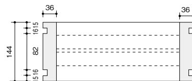
障子用・襖用(2×4工法用) (単位:mm)
