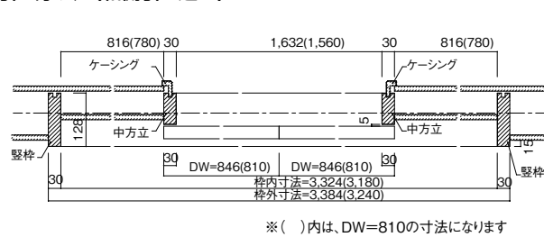
引き分け戸(和側引き込み) (単位:mm)
