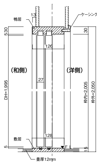
畳厚12mmご使用時(バリアフリー対応)敷居厚15mmタイプ
