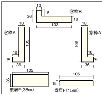
●在来工法用(窓枠幅105mm用)寸法図(mm)
