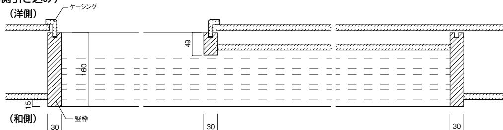
3枚引き込み戸(和側引き込み)
