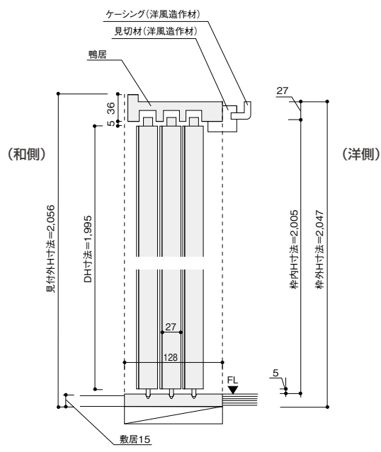
畳厚12mmご使用時(バリアフリー対応)敷居厚15mmタイプ
