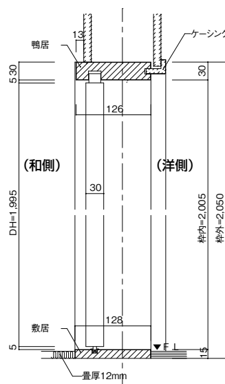
畳厚12mmご使用時(バリアフリー対応)敷居厚15mmタイプ (単位:mm)
