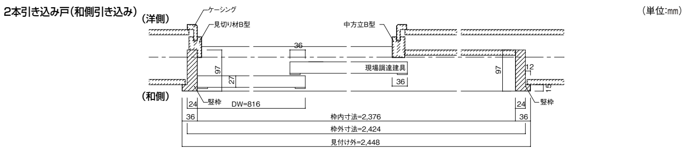
横断面図
