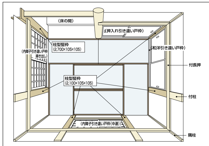
柱型竖枳使用例
