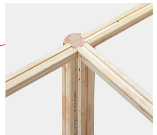
壁下地材との取り付け
