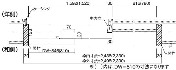
2枚引き込み戸(和側引き込み)
