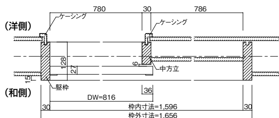
片引き戸(和側引き込み)
