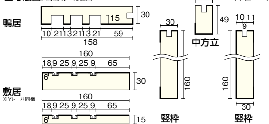
■寸法図 太線部分は化粧面
