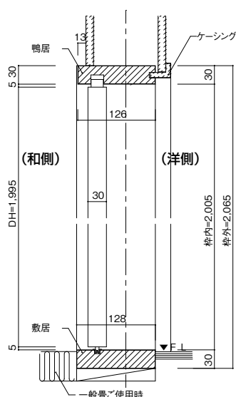
一般畳ご使用時(バリアフリー対応)敷居厚30mmタイプ (単位:mm)
