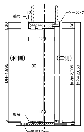
畳厚12mmご使用时(バリアフリー対応)敷居厚15mmタイプ
