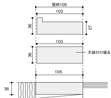
押し入れ開き戸枠セット
