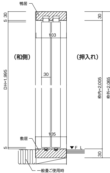
一般畳で使用时(バリアフリー対応)敷居厚30mmタイプ
