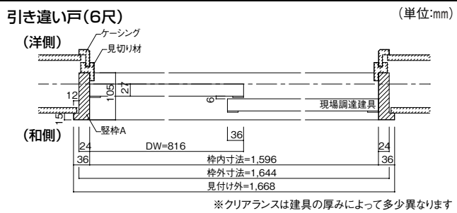
横断面図
