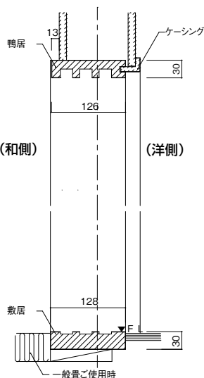
一般畳ご使用时(バリアフリー対応)敷居厚30mmタイプ
