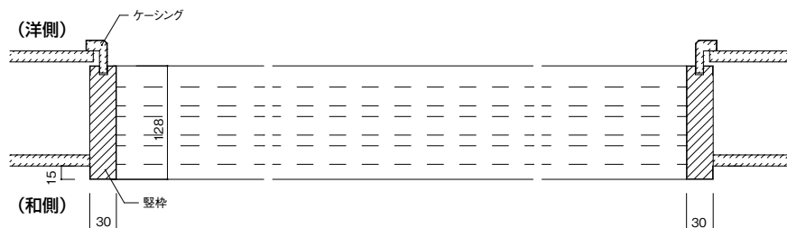
引き違い戸(3本引き)
