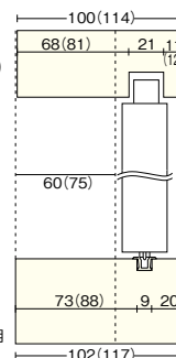
■真壁用 片引き戸 納まり図寸法図(mm)
