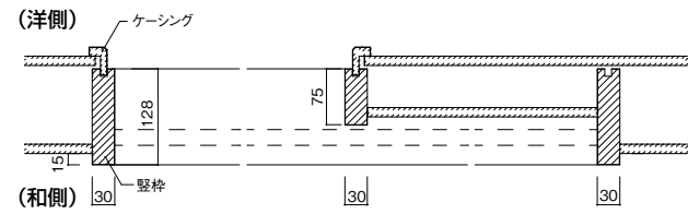
片引き戸(和側引き込み)
