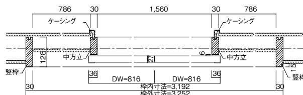
引き分け戸(和側引き込み)
