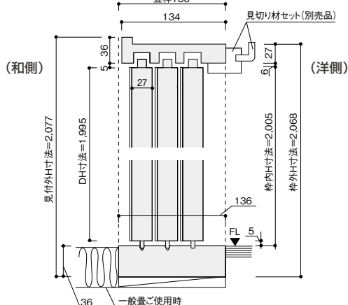
堅栓136 (単位: mm)
