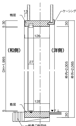
一般畳ご使用时(バリアフリー対応)敷居厚30mmタイプ
