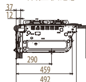
【A+39設置状態】
