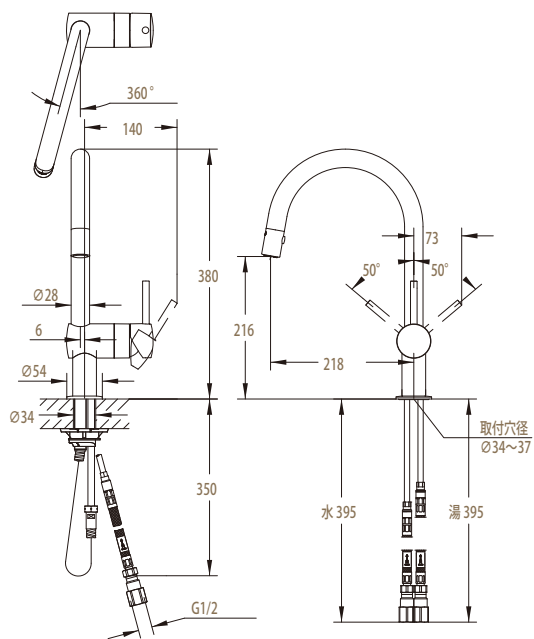
品番 HDFG007-HH 機種名 31095000W0
