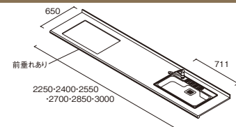
[ワイドスペーススタイル]
