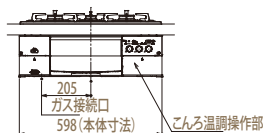
【正面図】
