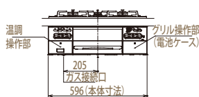
【正面図】
