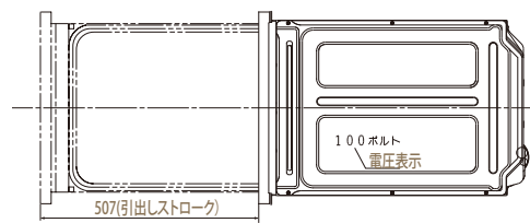
【平面図】
