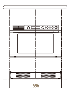
【正面図】
