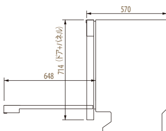
【側面図】
