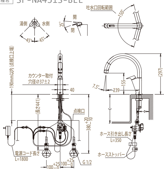
品番 HDFI003-GH 機種名 SF-NA451S-BEL
