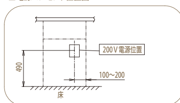
◎高さ調節寸法
