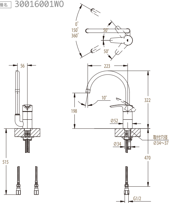
品番 HDFG008-GH 機種名 30016001W0
