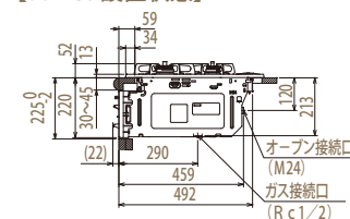
【A+37設置状態】
