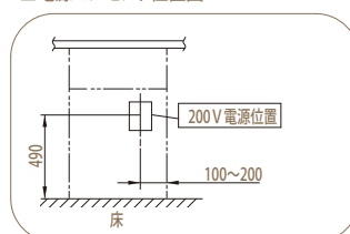
■電源コンセント位置図
