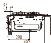
【A+39設置状態】
