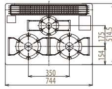
【側面図】
