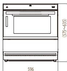
【正面図】
