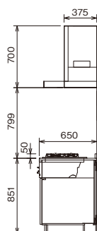
■レンジフード側断面図
