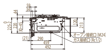
【側面図】 【A+59設置状態】
