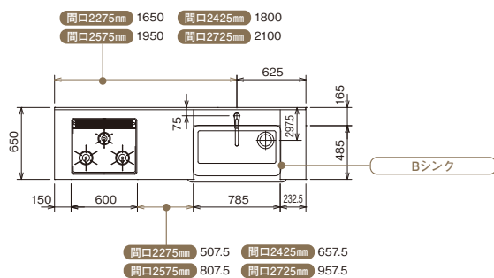
■ワークトップ俯瞰図 (本図はクォーツストーン×Bシンクの場合)
