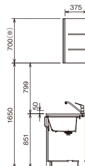
■キャビネット側断面図
