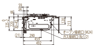
【側面図】 【A+59設置状態】
