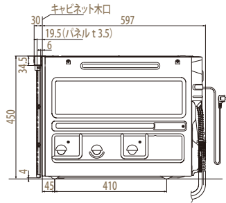
【側面図】
