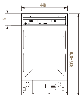
【正面図】
