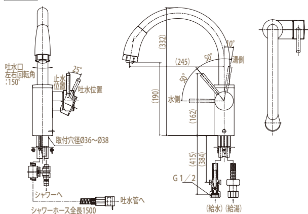
品番 HDFK008-HH 機種名 KM708GW0
