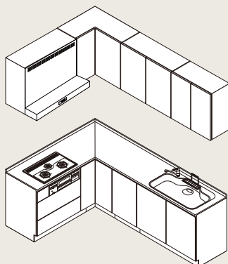
L型プラン
