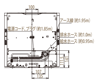
【背面図】
