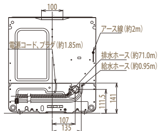
【背面図】
