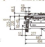
【A+59設置状態】
