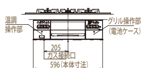
【正面図】
