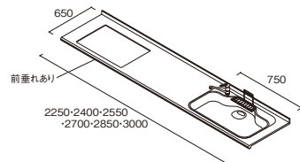
[ワイドスペーススタイル]
