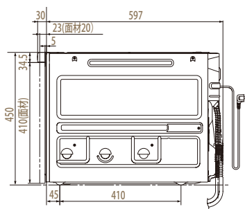
【背面図】
