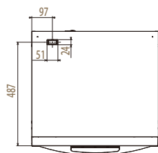
【天面図】
