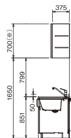
■キャビネット側断面図
