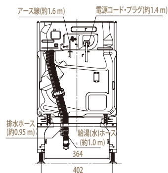
【背面図】
