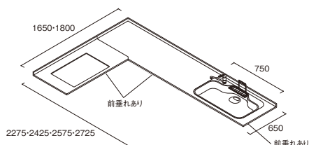
[ワイドスペーススタイル]
